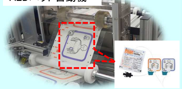
AEDパッド自動機
